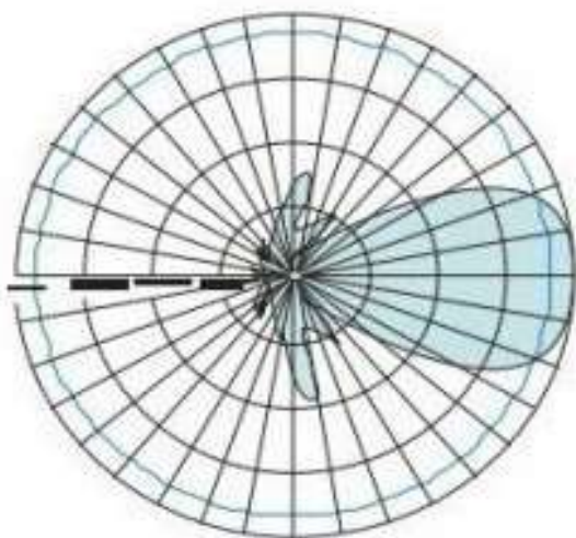
E-plane
